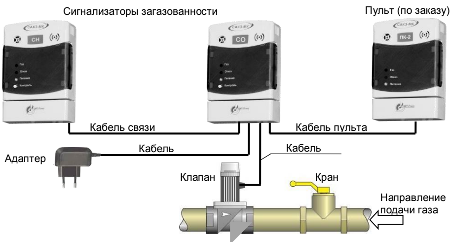
Рисунок 1 - Структурно-функциональная схема стандартной системы
